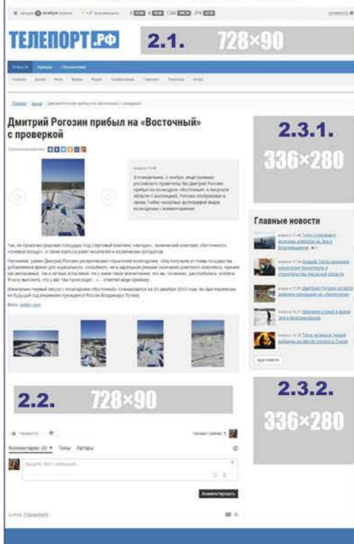
Рис. 2. Страницы новостей
