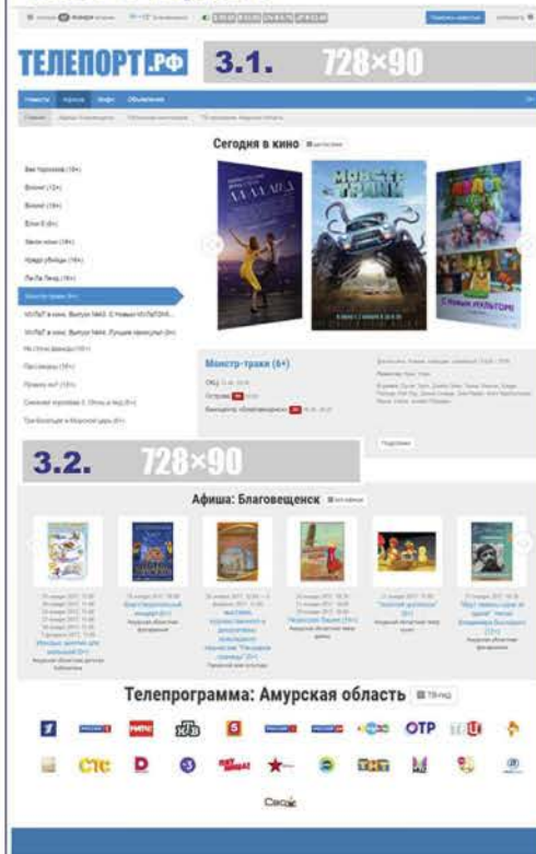
Рис. 3. Афиша
